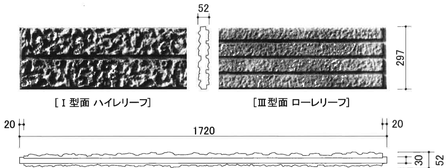
DECO板 I・III 型 [両面/レリーフ]
