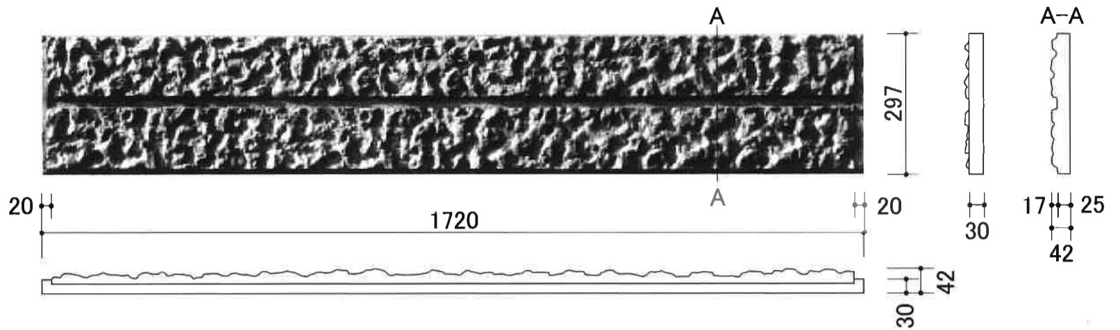
DECO板 I 型 [片面/ハイレリーフ]
