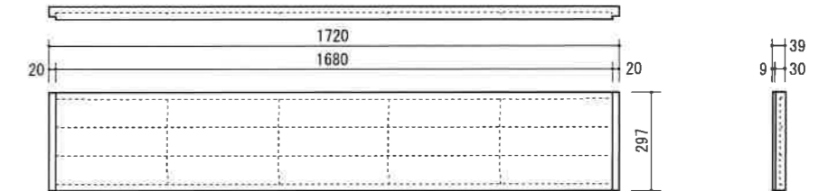
幅木 [JIS]
