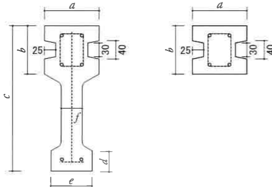
控付柱 B-B 断面
