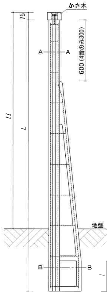
控付柱
