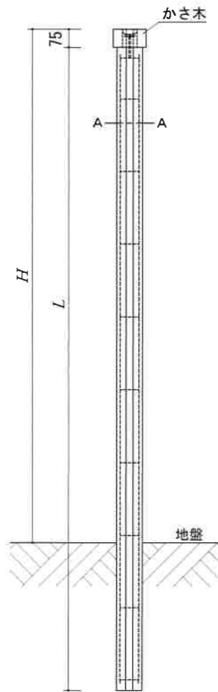
柱(直柱)
