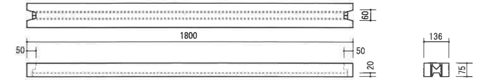
かさ木 [JIS]
