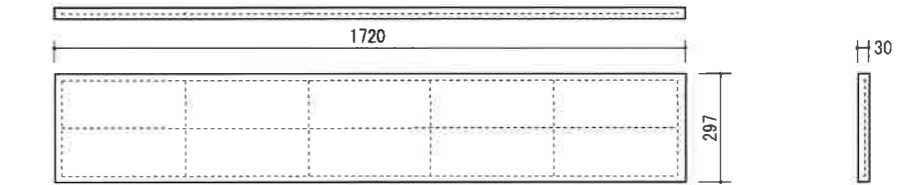
板 [JIS]
